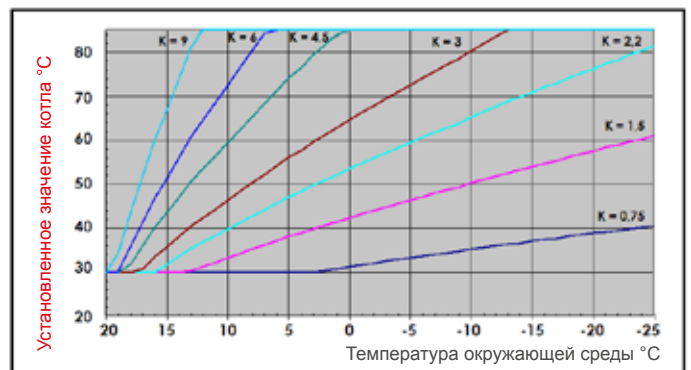
Рисунок 33. Кривая эксплуатации внешнего датчика температуры
