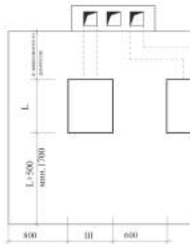
Рис. 15. Планировка котельной.
