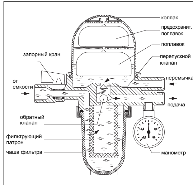
Принципиальная схема
