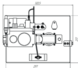
Рис. 5 Габариты горелки АГГ-40К (2015)
