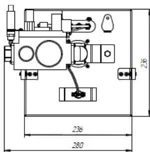
Рис. 4 Габариты горелок АГГ-13К; АГГ-26К
