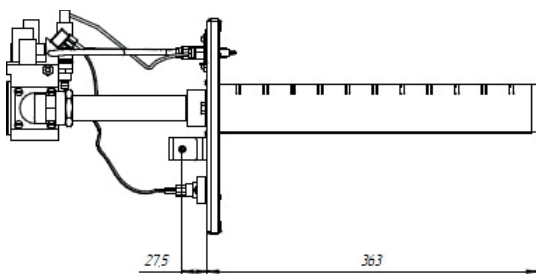
Рис. 4 Габариты горелок АГГ-13К; АГГ-26К
