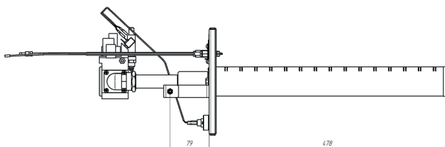
Рис. 5 Габариты горелки АГГ-40К (2015)
