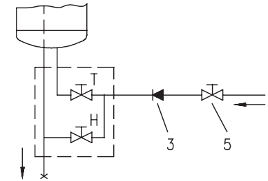
Das Durchflußsystem
