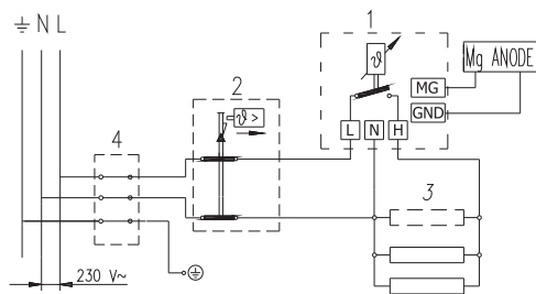
Elektroschema
