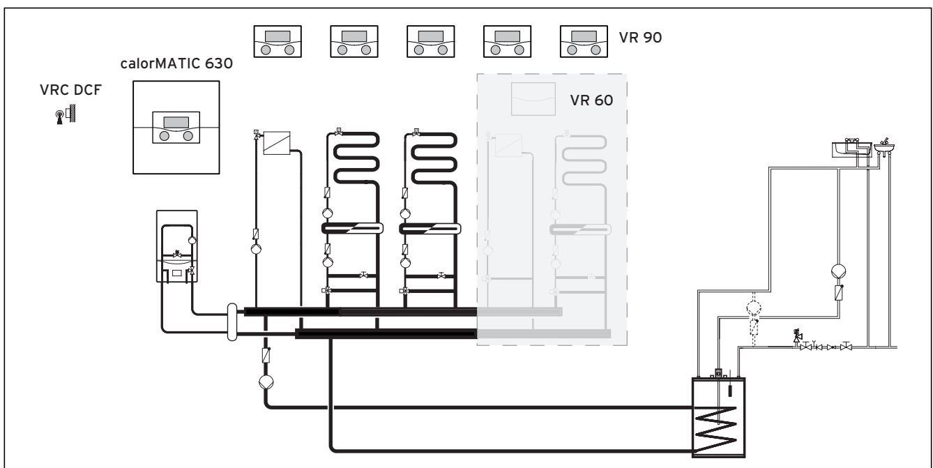
Рис. 3.1 Обзор системы
