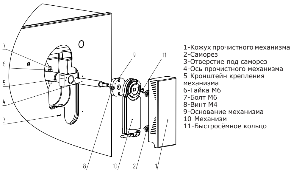
Рис.3 Установка механизма чистки теплообменника
