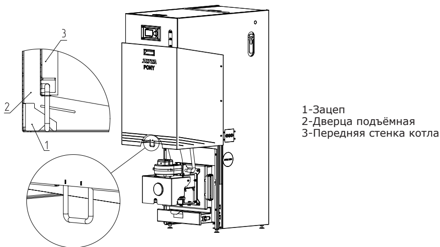
Рис.2 Зацеп двери
