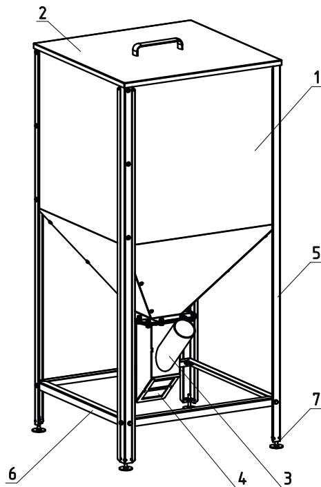
Рис.4 Топливный бункер
