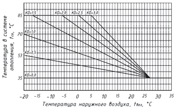
Рис. 9. Кривые нагрева
