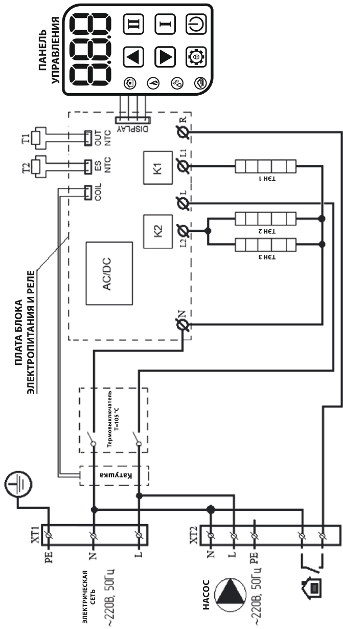
Рисунок 5.7. Схема электрическая принципиальная котлов ЕСО-3, ЕСО-4,5 (220В) T1 - датчик температуры котла, T2 - датчик температуры воздуха в комнате, K1, K2 - реле, - комнатный термостат
