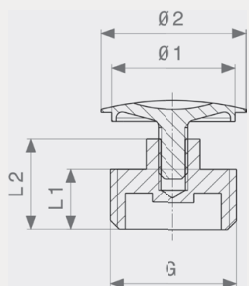
Заглушка - латунь Модель 1752
