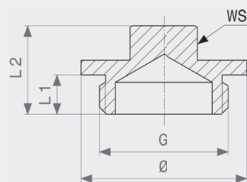
Заглушка - латунь Модель 1751
