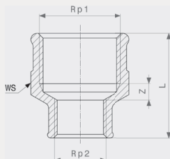
Редукционная муфта - бронза Модель 3240
