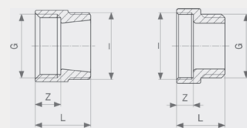
Ниппель-переход - бронза Модель 3252
