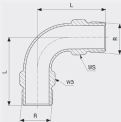
Отвод 90° - бронза Модель 3003
