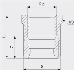
Ниппель-переход - бронза Модель 3243
