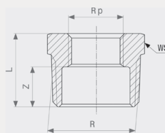
Редукционная вставка - бронза Модель 3241
