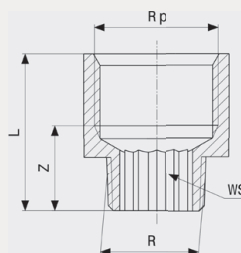
Редукционная вставка - бронза Модель 3242
