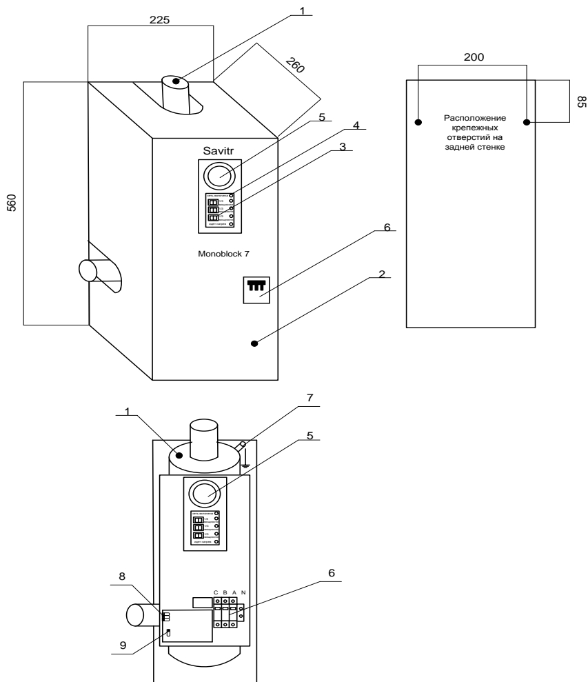
Рис.1 Общий вид изделия типа «Monoblock».
