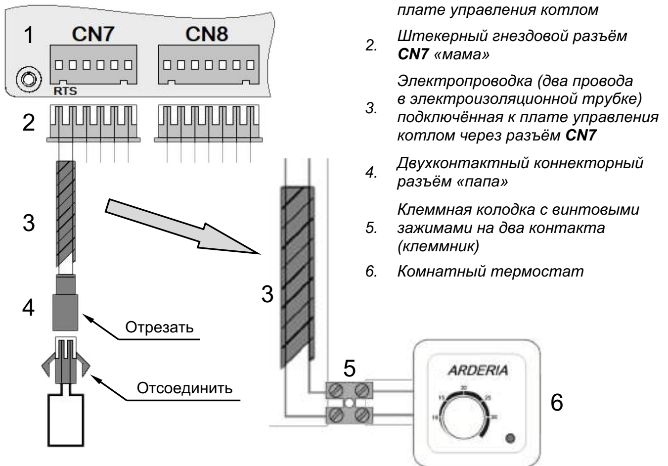
Рис. 49 Принципиальная схема подключения комнатного термостата непосредственно к электропроводке (двум проводам в электроизоляционной трубке) присоединённой к плате управления котлом через разъём CN7.
