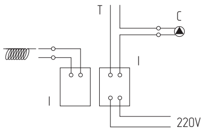
Электрическая схема WHU900–WHU1100
