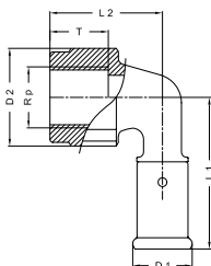
ТИП: 6PK Угол переходной, пресс-внутренняя резьба
