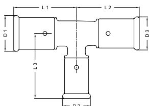
ТИП: 11PKG Тройник переходной с двух сторон
