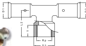
ТИП: 13P Тройник переходной, пресс-внутренняя резьба
