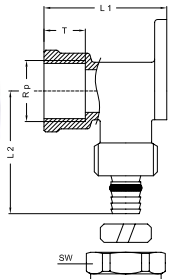
ТИП: H Монтажная пластина для водорозеток
