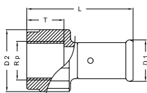
ТИП: 18PKG Муфта переходная, пресс- внутренняя резьба
