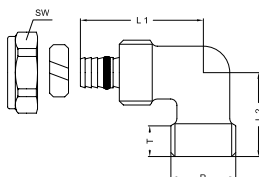
ТИП: 5 Угол переходной, обжим- внешняя резьба
