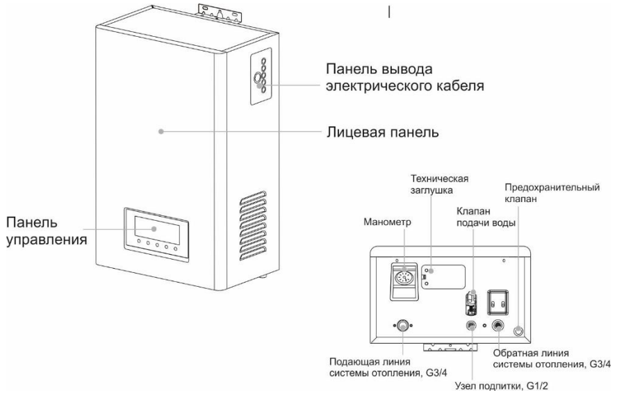
Рис. 1. Конструкция изделия
