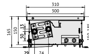
Разрез Qtherm НК2 310.150 с U-образным бортом.
