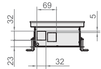
Разрез Qtherm НК Mini с U-образным бортом.
