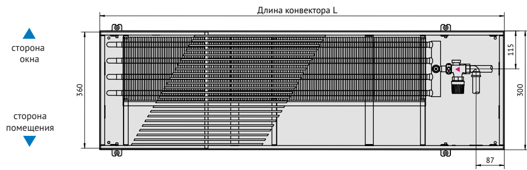
Вид сверху конвектора Ntherm Maxi 370 с роликовой решеткой, с U-образным бортом.
