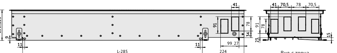
Вид с торца Qtherm НК4 310.150 с F-образным бортом.
