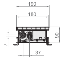
Вид с торца Qtherm НК Mini с U-образным бортом.
