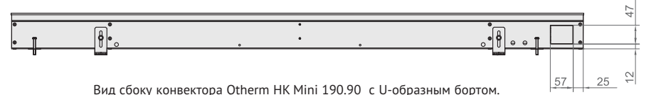
Вид сбоку конвектора Qtherm НК Mini 190.90 с U-образным бортом.
