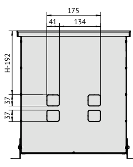
Вид с торца Ntherm Maxi 370 с U-образным бортом.
