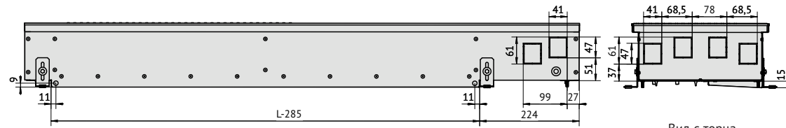
Вид сбоку конвектора Qtherm НК2 310.130 с U-образным бортом.
