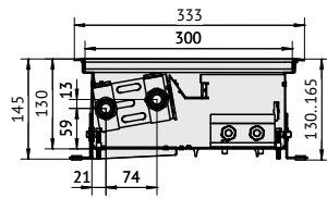
Разрез Qtherm НК4 310.130 с F-образным бортом.
