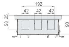
Вид с торца Qtherm ECO 275 с U-образным бортом.
