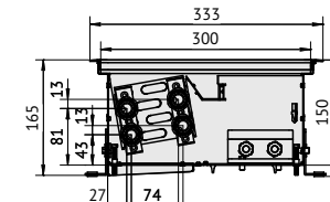
Разрез Qtherm НК4 310.150 с F-образным бортом.
