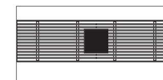
Вырез под колонну в середине конвектора
