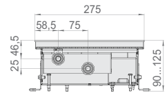
Разрез Qtherm ECO 275 с U-образным бортом.
