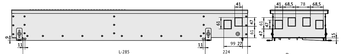
Вид с торца Qtherm НК2 310.150 с U-образным бортом.
