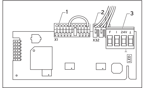
Şekil. 3.4 Kablo bağlantıları (soketli X1)
