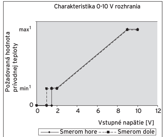
Obr. 3.2 Charakteristika rozhrania 0-10 V s požadovanou hodnotou prívodnej teploty
